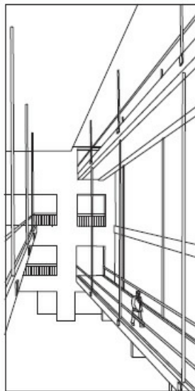
El diseño propuesto para la pasarela. A la derecha, las pasarelas del segundo y cuarto piso que se derrumbaron están suspendidas por los mismos tirantes.
